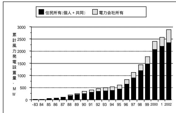
デンマークにおける風力発電の所有者別設備容量の推移 (Danish Wind Industry Association, 2004)
